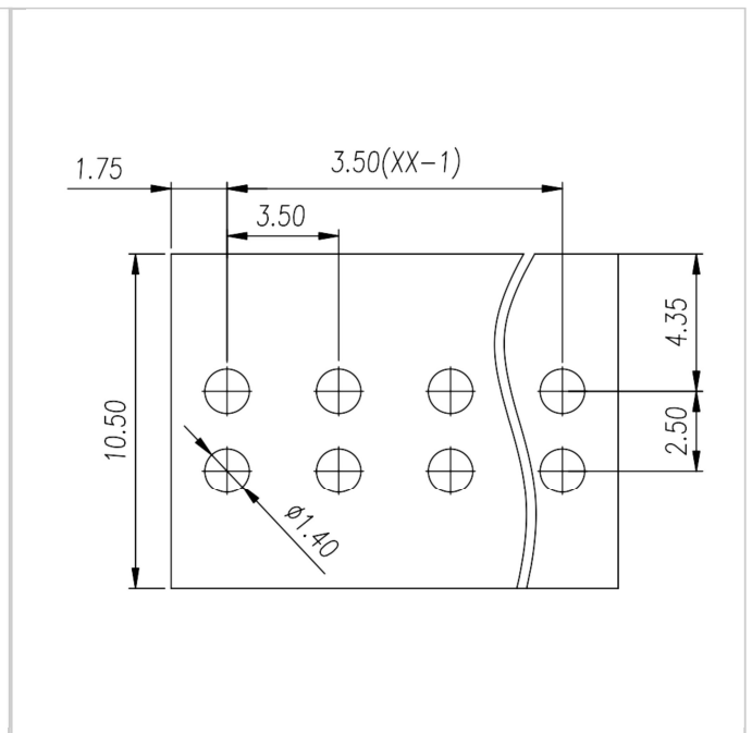
PCB开孔图
